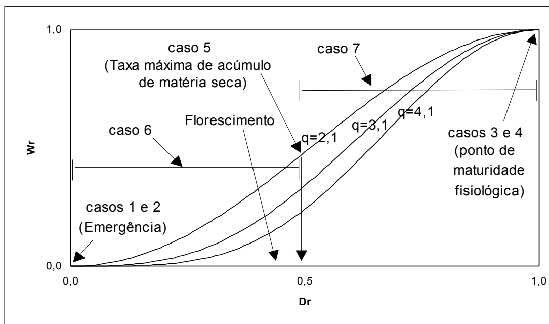
Figura 1 - Modelo do cosseno para três diferentes fatores de forma (q) especificando os sete diferentes casos.
