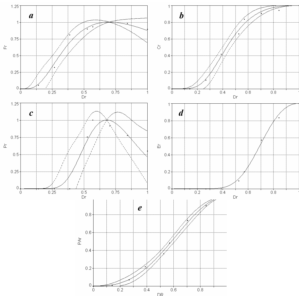
Figura 2 - Valores médios observados e estimados de matéria seca relativa de (a) folha (Fr) (modelo universal tipo II); (b) colmo (Cr) (modelo universal tipo I); (c) pendão (Pr) (modelo universal tipo II); (d) espiga (Er) (modelo universal tipo I) e (e) parte aérea (PAR) (modelo universal tipo I) em função do desenvolvimento relativo (Dr) da cultura de milho. As curvas externas (inferior e superior) ilustram o intervalo de confiança com 99% de probabilidade.
